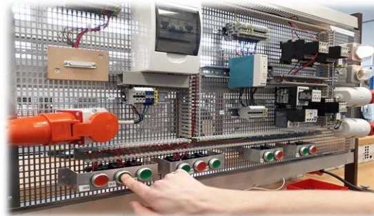
Aufbau einer Steuerung mit Schützen
