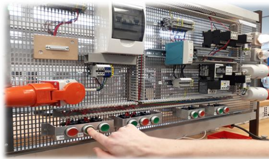
Aufbau einer Steuerung mit Schützen
